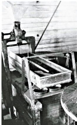
Säden rinner ned till kvarnstenarna, till höger en sikt.
